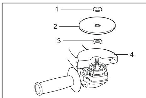
► 1. Контргайка 2. Абразивный отрезной диск/ алмазный диск 3. Внутренний фланец 4. Защитный кожух для абразивного отрезного диска/алмазного диска
