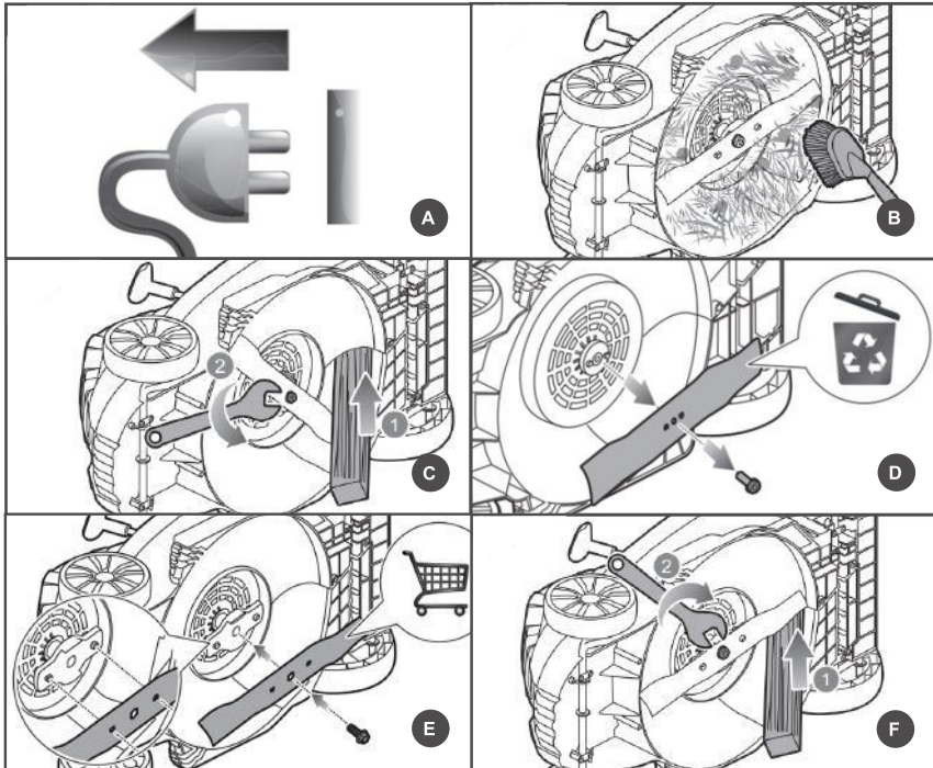
Рис. 17 Замена ножа
