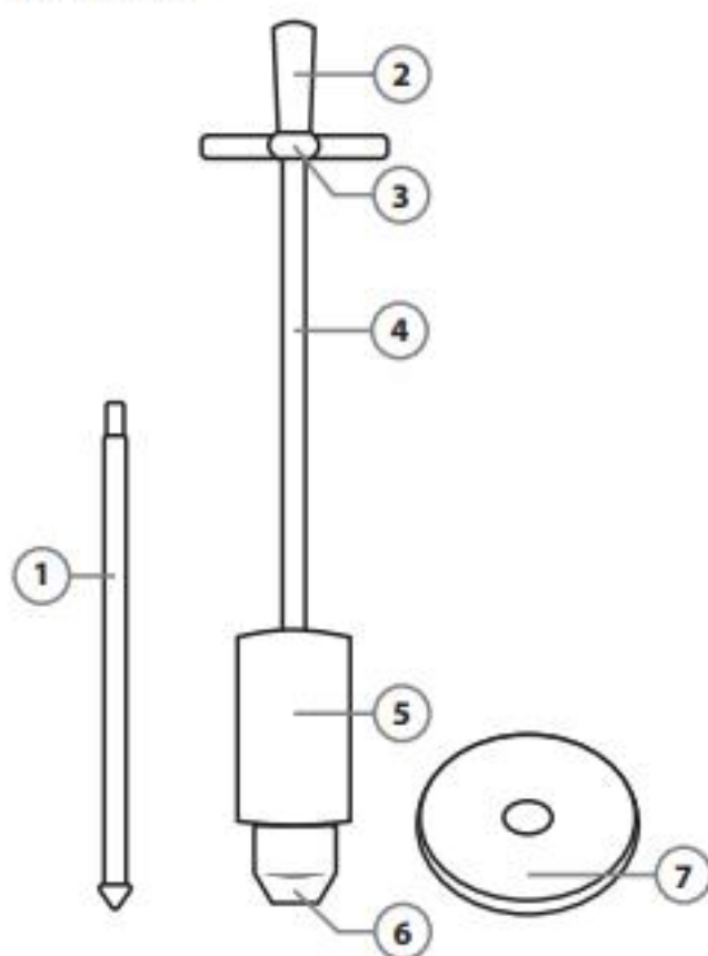
Рис.1 Общий вид прибора
